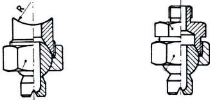
3. Kugel-Düsen max. 20 bar (Seite 2.10)
