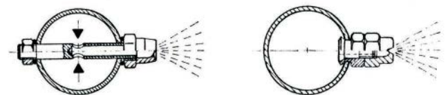
10. Hohlspindel-Düsen H für Rechteck- und Rundrohre, max. 10 bar Klemmring U für Rechteck und Rundrohre, max. 4 bar (Seite 8.13 und 8.14)
