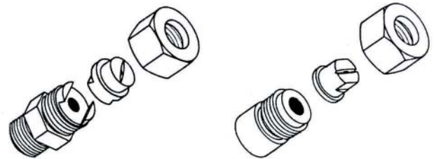
4. Düsenmundstücke mit und ohne Schwalbenschwanz Hochdruck (Kapitel 7)
