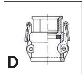
Mutterteil/ Innengewinde
