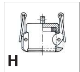
Mutterteil/ Stopfen
