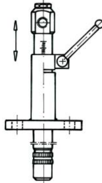
Düsen-Lanze mit Schiebehülse und Flansch nach Wahl, Standard 120 mm Ø
