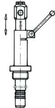
Düsen-Lanze mit Schiebehülse und Kopfgewinde, auf Anfrage
