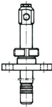
Düsen-Lanze mit Verschraubung, starr oder verschiebbar DIN 11851 bzw. DIN 11864-1
