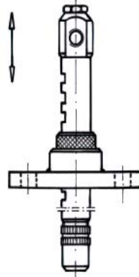
Düsen-Lanze mit integrierter Höhenjustierung mittels klemmbarer Einstellscheibe, kompatibel zu Systemen auf dem Markt
