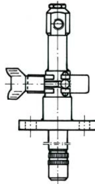
Düsen-Lanze mit stabiler Klammer und Clampstutzen, starr oder mit Schiebehülse
