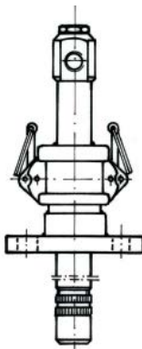
Düsen-Lanze mit Camlocverschluss, starr oder mit kombinierter Schiebehülse
